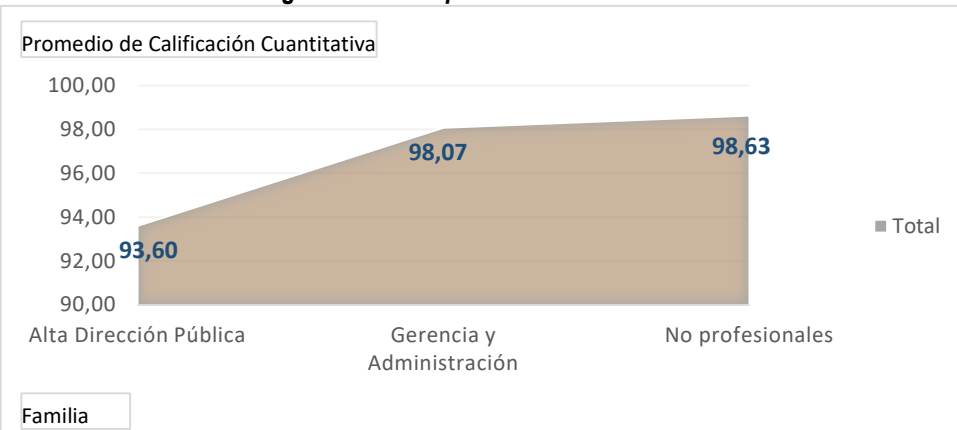
Gráfico 3: Resultados según familia de puestos
